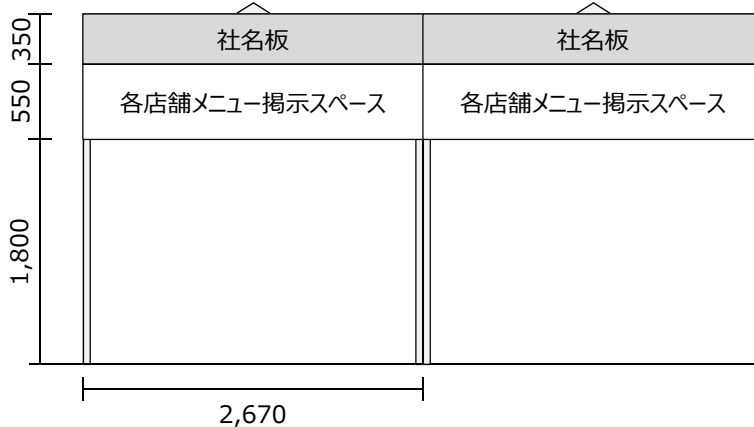
◎ 立面図 (PLAN③)
