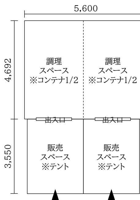
◎平面図(PLAN③)
