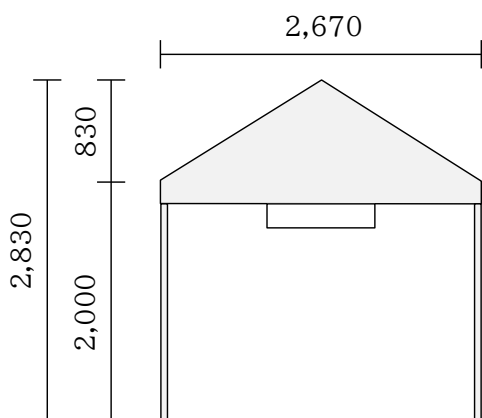
◎立面図(PLAN①・PLAN②共通)
